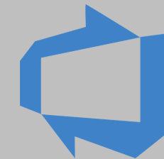
Azure DevOps
